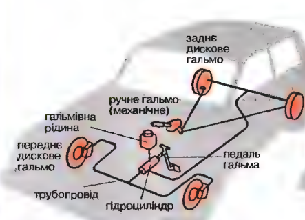
Система гальмування
